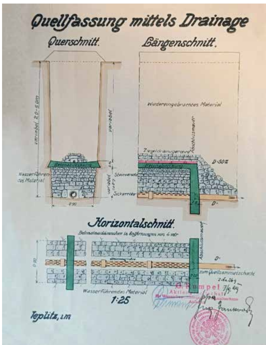
Projekt zachycení vodního zdroje pomocí drenáže
